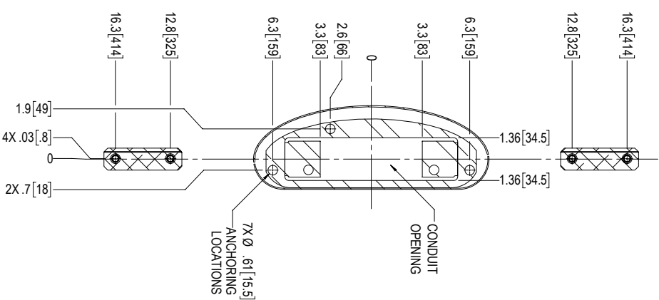
SU4500 SECTION A-A (DO NOT SCALE)
