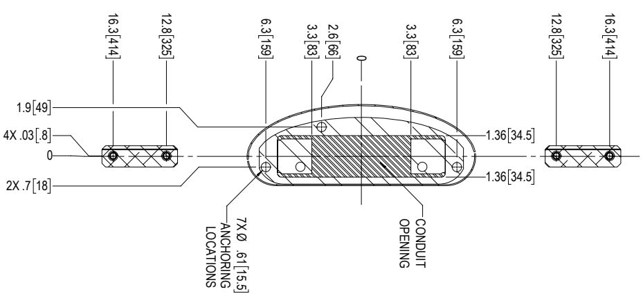
SU4500 SECTION A-A (DO NOT SCALE)
